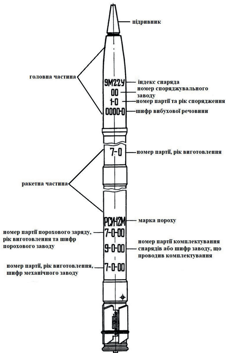
Рис. 2. Схема снаряда 122-мм до РСЗВ «Град».
