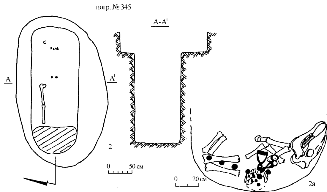
Рис. 3. Захоронения с конём II типа: 1 – погребение № 413, 2 – погребение № 345; 2а – расположение конских останков в погр. № 345.
