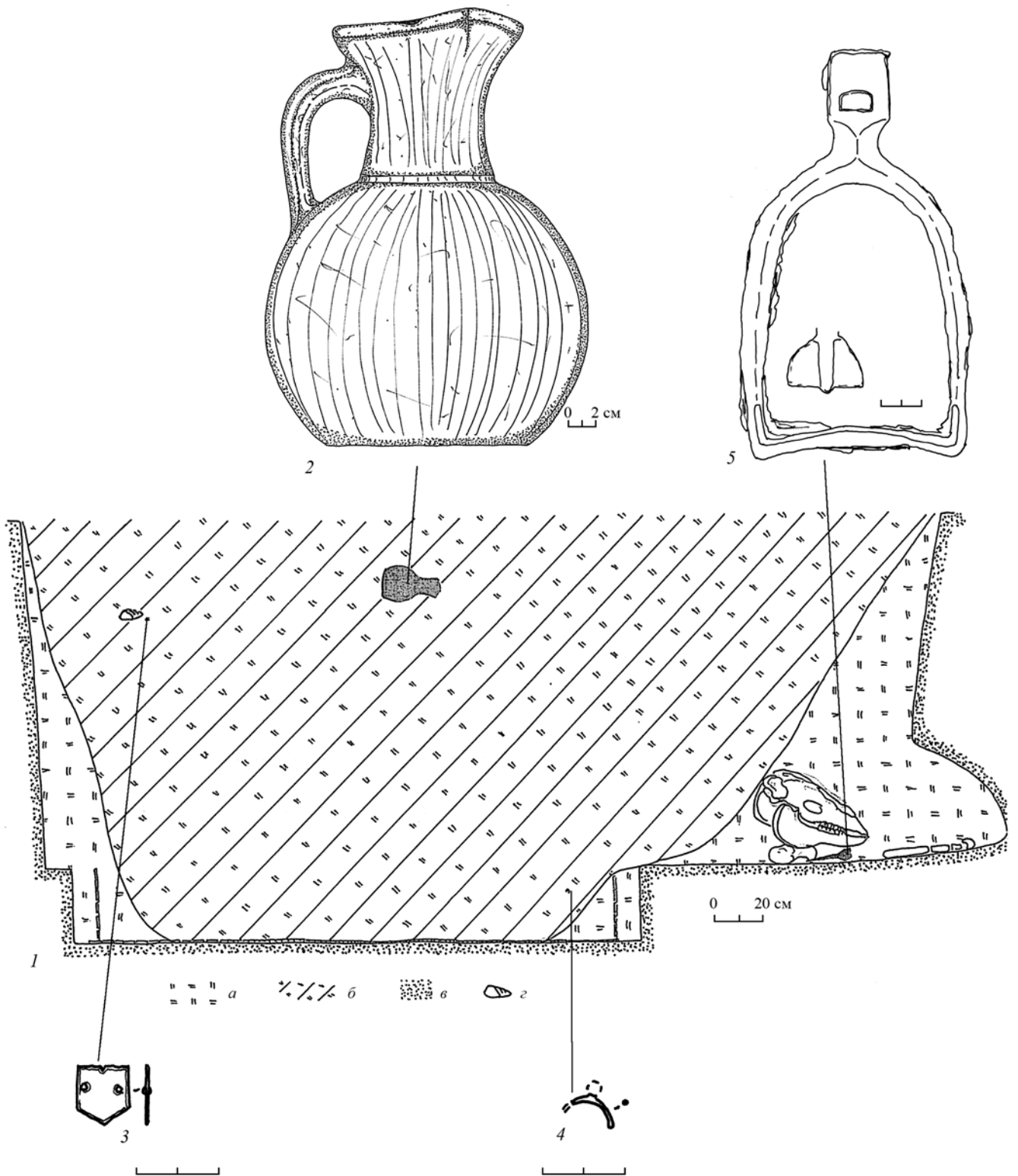
Рис. 6. Погребение № 527. Разрез заполнения могильной ямы и находки: 1 – продольный разрез заполнения, 2 – кувшин, 3 – бляшка от ремней оголовья, 4 – фрагмент кольца сережки, 5 – стремя (2 – глина, 3, 4 – серебро, 5 – железо). Условные обозначения: а – первоначальное заполнение могильной ямы (светло-серый песчаный грунт), б – заполнение позднейшего вкопа (слоистая темно-серая супесь), в – материк (светло-желтый песок), z – крестцовая кость лошади.
