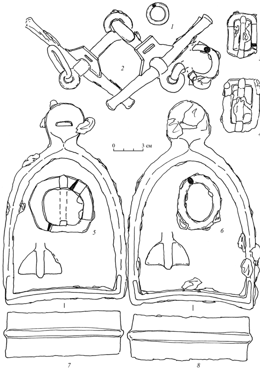
Рис. 4. Элементы конского снаряжения из погребения № 529: 1, 6 – сбруйные кольца, 2 – удила, 3–5 – сбруйные пряжки, 7, 8 – стремяна (1 – бронза, 2–8 – железо).
