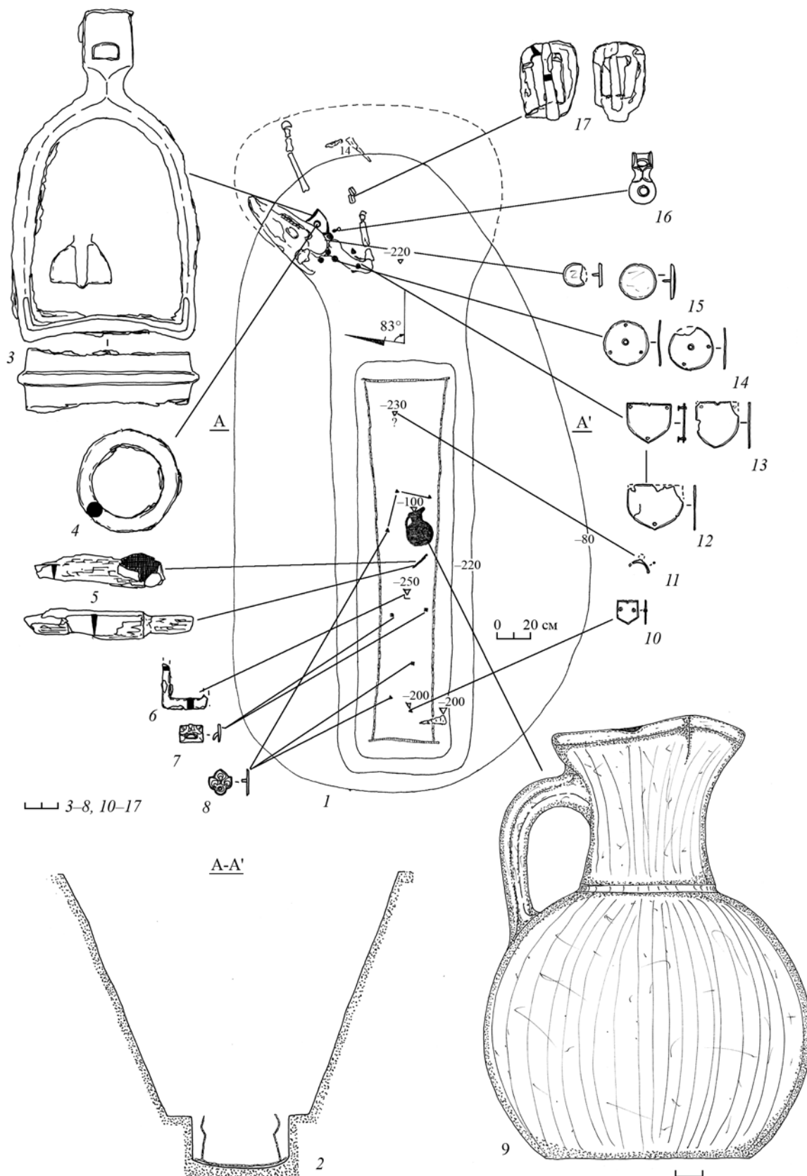
Рис. 7. Погребение № 527. План, разрез и находки: 1 – план погребения, 2 – поперечный разрез погребения, 3 – стрема, 4 – сбруйное кольцо, 5 – ножи, 6 – фрагмент поясной пряжки, 7, 8 – поясные бляшки, 9 – кувшин, 10 – бляшка от ремней оголовья, 11 – фрагмент кольца сережки, 12–14 – фалары, 15 – бляшки от ремней оголовья, 16 – чумбурный блок, 17 – сбруйные пряжки (3–6, 17 – железо, 7, 8, 10–15 – серебро, 9 – глина, 16 – бронза).
