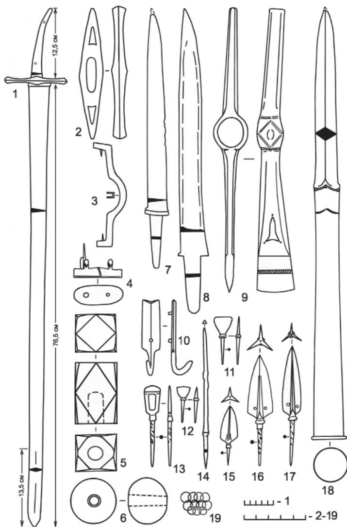
Рис. 5. Предметы вооружения, про- рисовка (все – железо). Fig. 5. Armament, drawing (all – iron).
